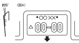
ナンバープレートが約5°前傾し、約18mm下がります。
